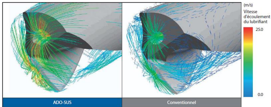
Analyse de l'écoulement du lubrifiant avec une vitesse de rotation de 2,200min-1
